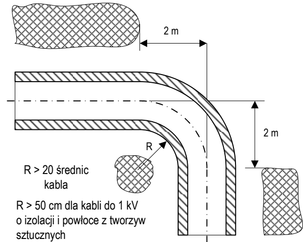
Promień łuku rowu kablowego w zależności od rodzaju kabla
