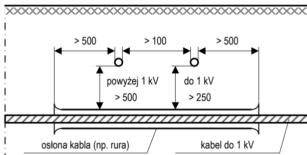
Odległości między kablami do 1 kV ułożonymi w ziemi
