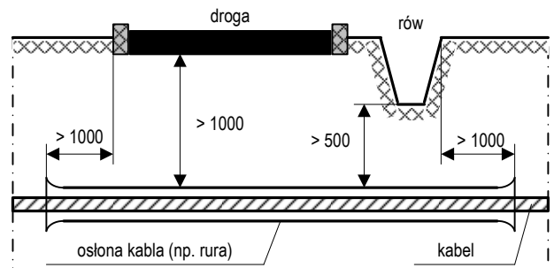
Odległości kabli ułożonych w ziemi pod drogami
